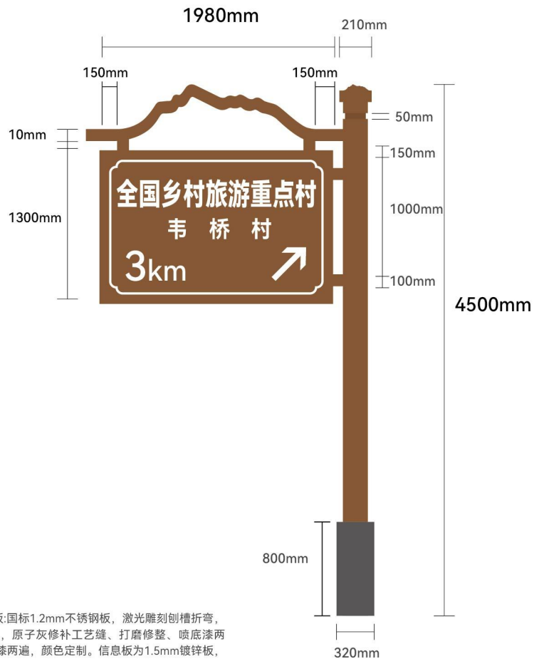
正视图
