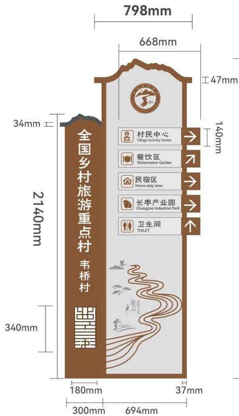
正视图
